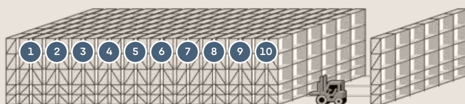
Soluzione compattabile Ipotesi di progetto Superficie occupata mq 687 Capacità bancali n. 2376
